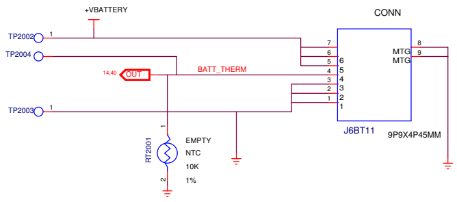
CON7_BAT_RCPT_CPL7506 H18079-001
