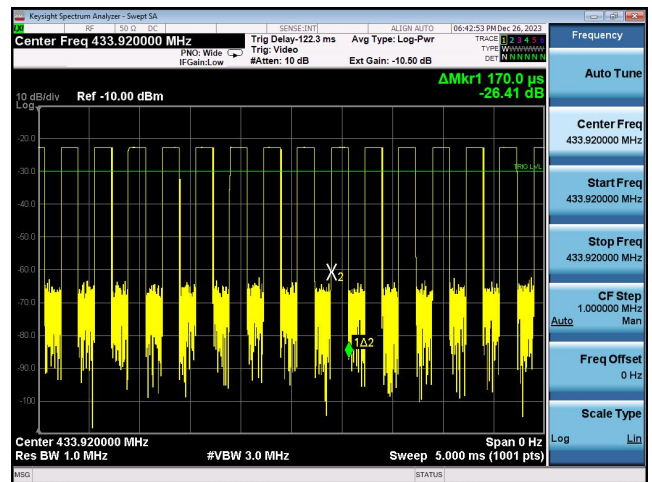
433.92 MHz: Burst 1
