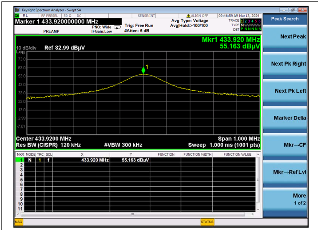
(Antenna Horizontal)
