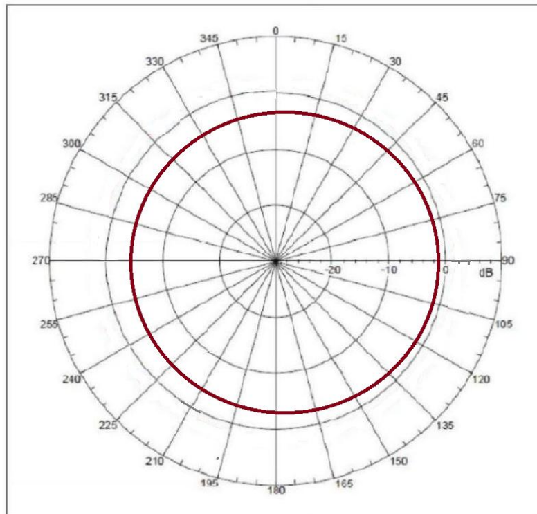
2420MHz
