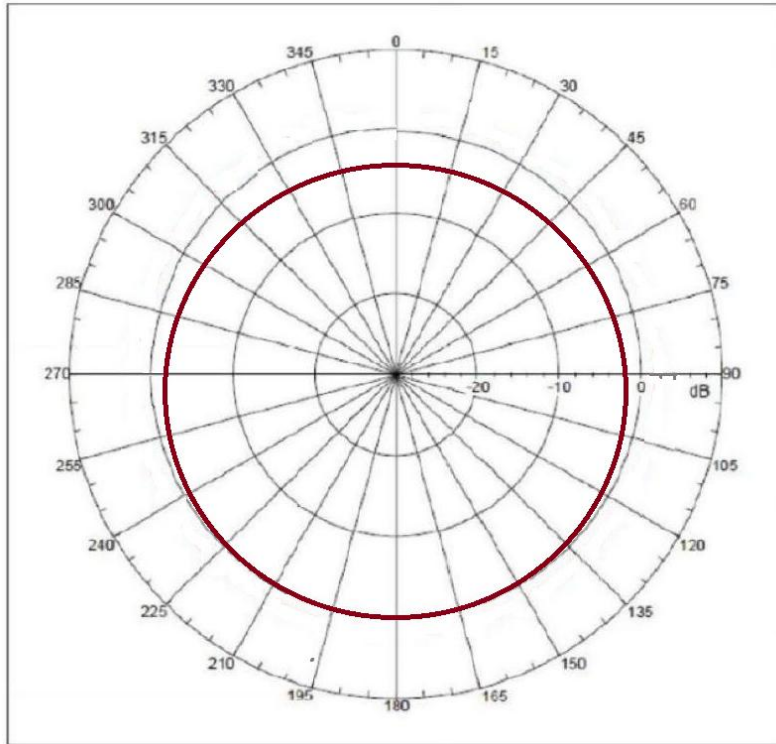
2480MHz
