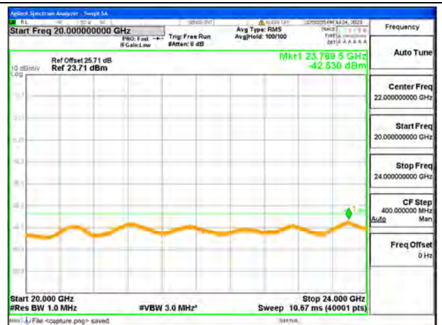
B30-20G-24G / 10MHz / High CH / QPSK
