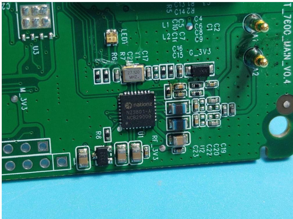
IC Chip 2
