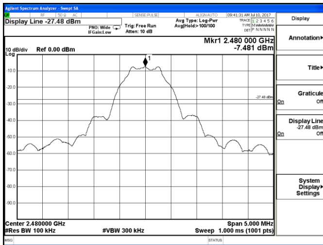
2479 – 2481 MHz
