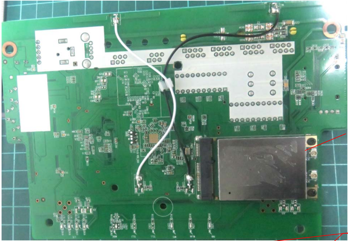
LTE module
