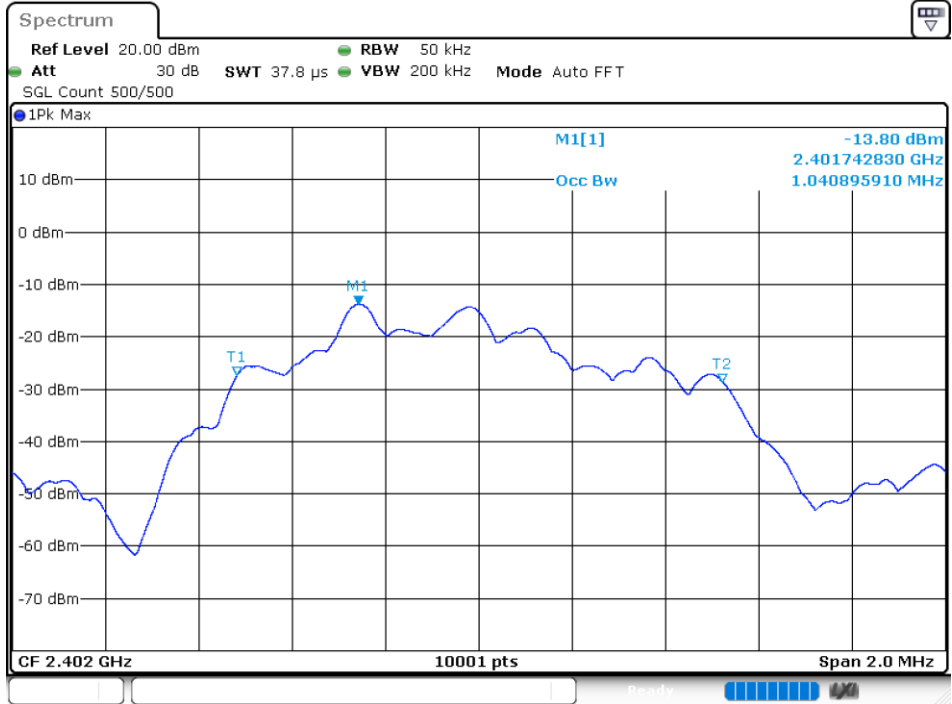
OBW NVNT GFSK 2402MHz Ant1
