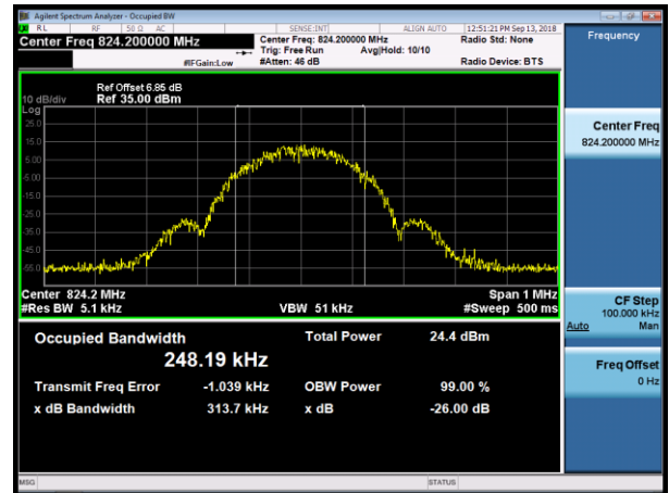
GSM 850-LCH-EDGE
