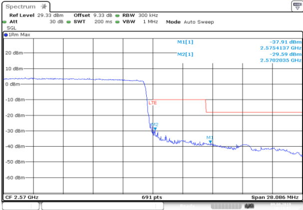
HCH_QPSK_75RB#0
