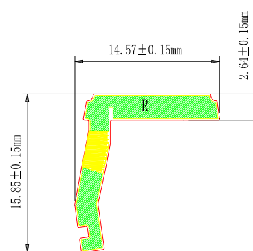
R 边天线尺寸图
