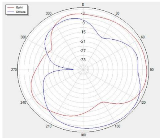
Theta=90 freq=2400MHz
