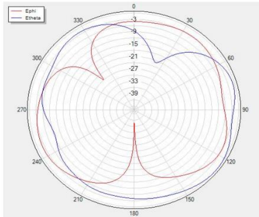
Theta=90 freq=2400MHz
