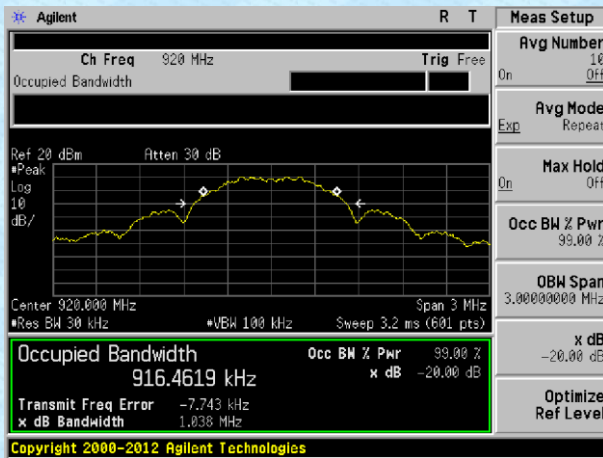
920MHz
