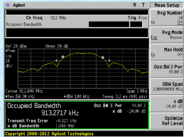
912MHz
