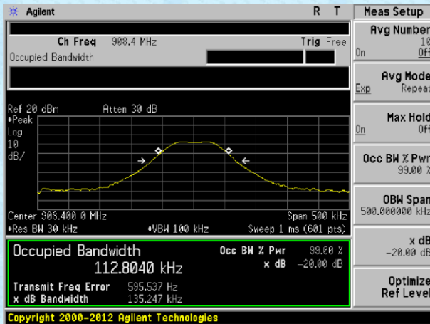
908.4MHz
