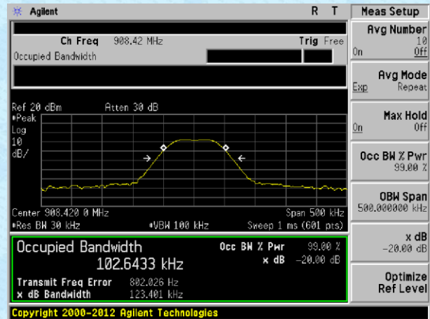
908.42MHz
