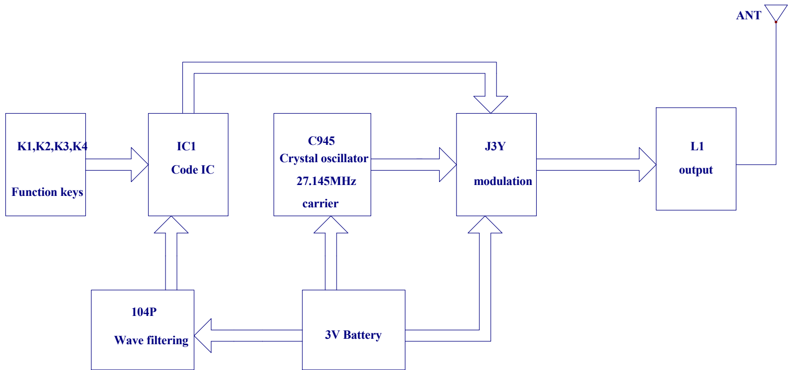
Signal flow 发射流程图
