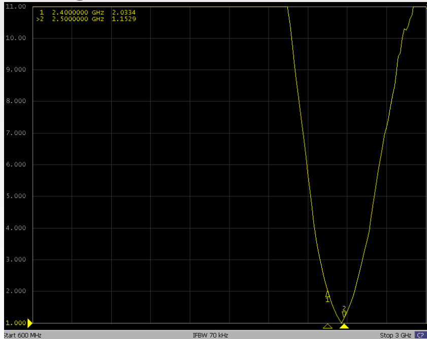
VSWR
