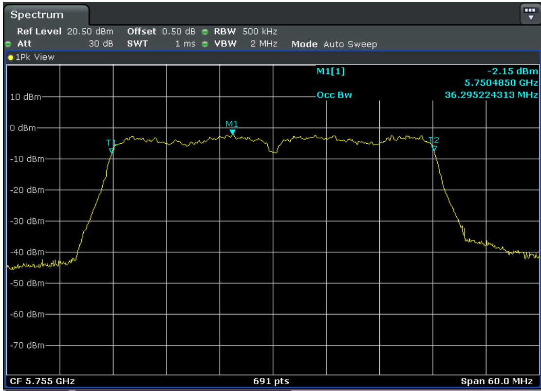
5755MHz-Ant2
