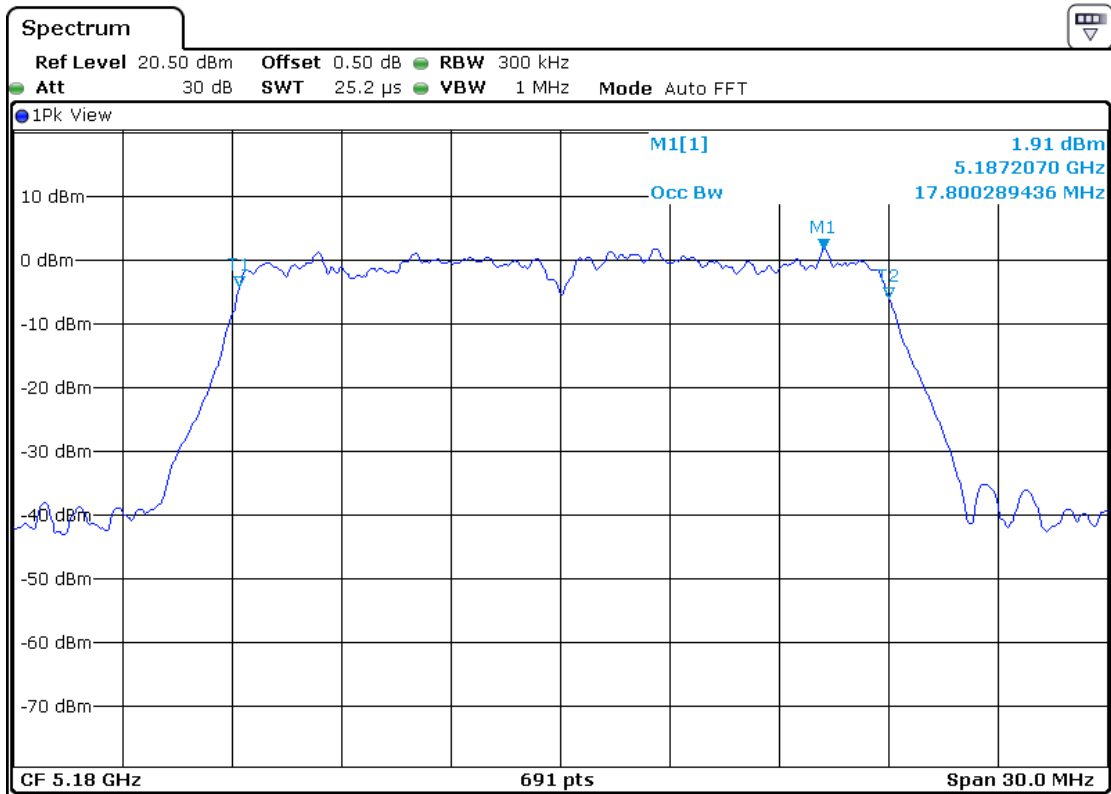
5180MHz-Ant2
