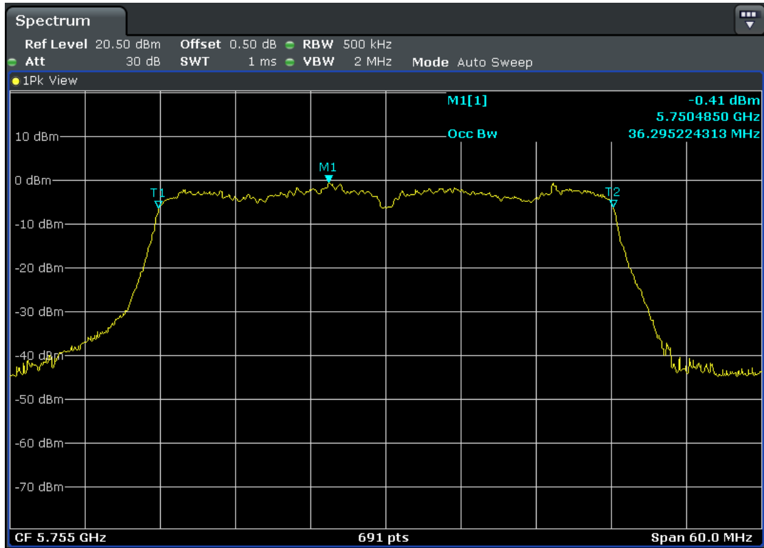
5755MHz-Ant2
