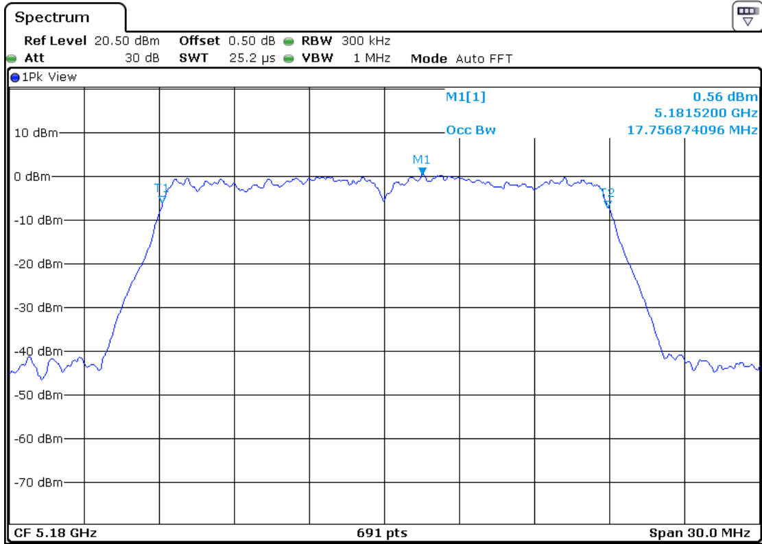
5180MHz-Ant2
