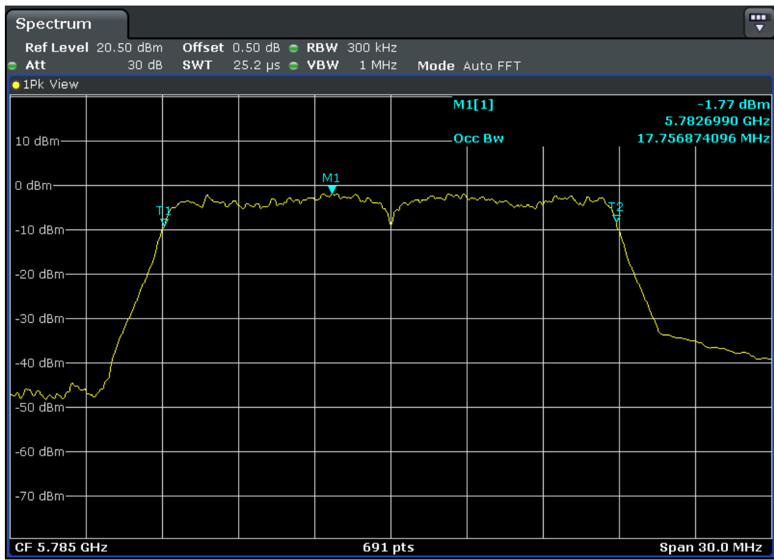
5785MHz-Ant2
