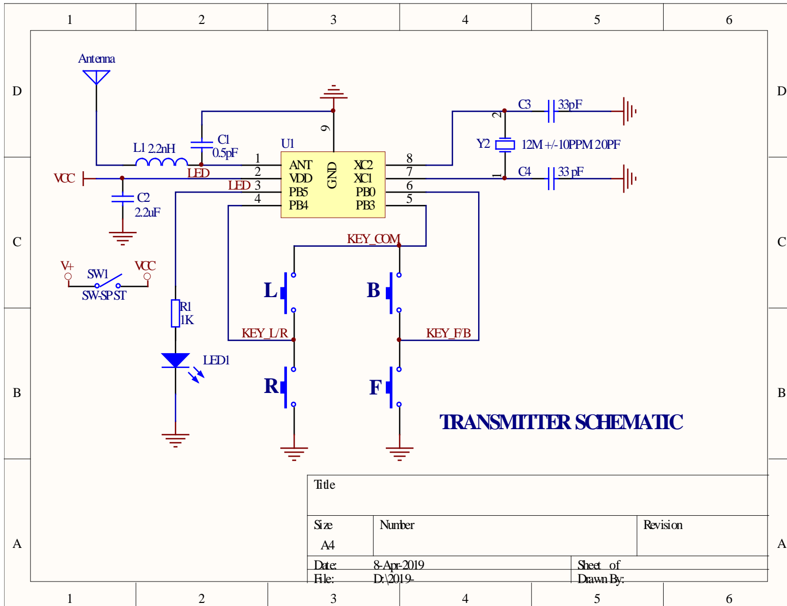
YX-2.4G-92T-Circuit diagram 发射板电路原理图
