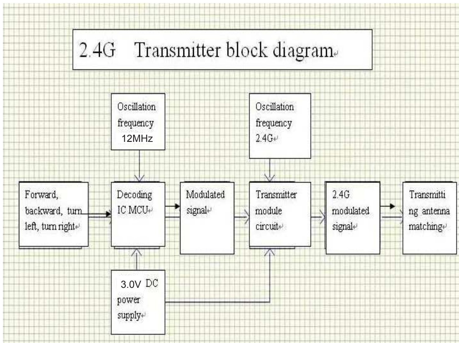
YX-2.4G-92T-PCB-Block diagram 发射板方框图
