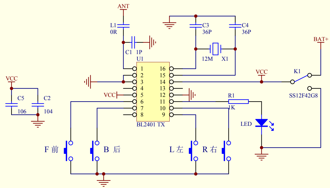
ZS-227ATX 原理图
