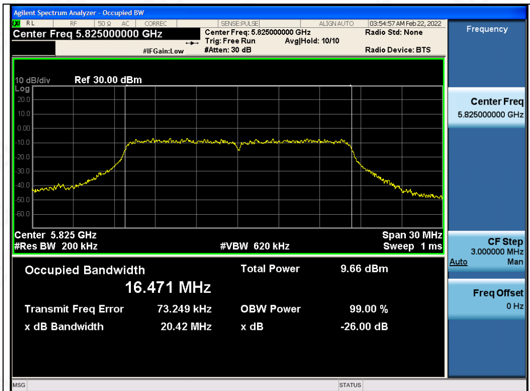
Test_Graph_802.11a_ANT1_5825_6Mbps_OBW
