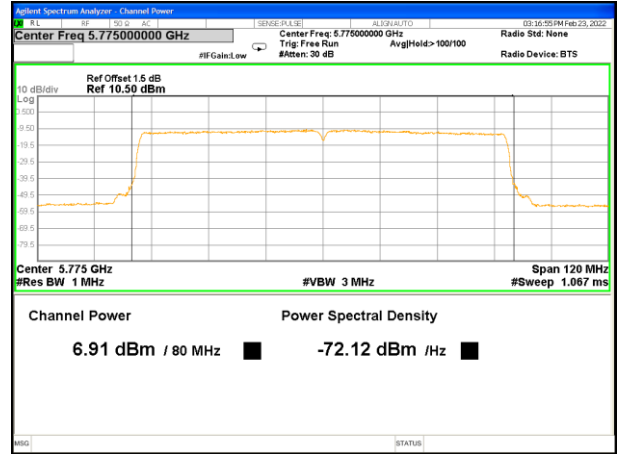
5775MHz_AV_Ant A
