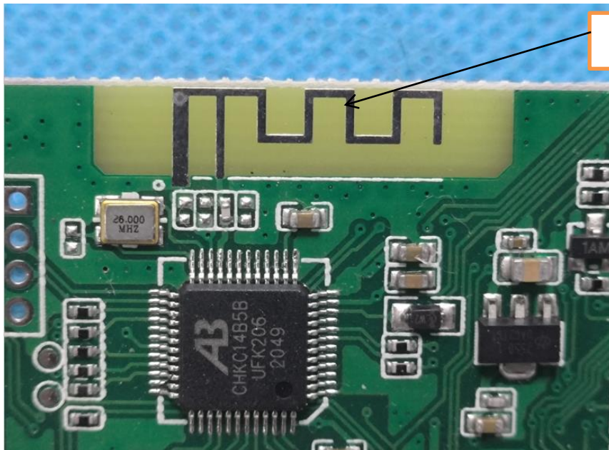
PCB ANT
