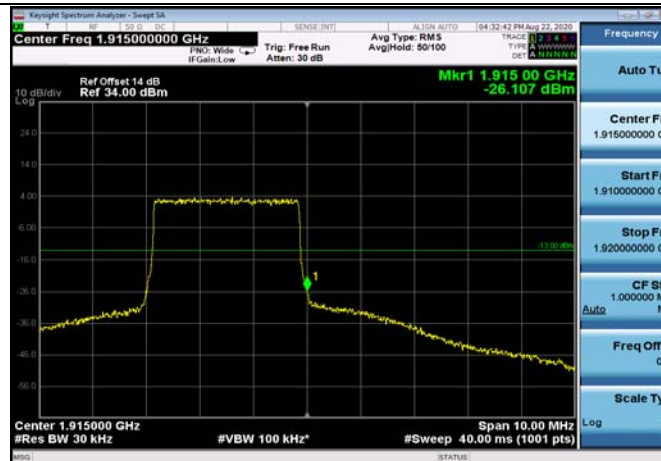
HighRange_FDD25_5MHz_1912.5_OneRB_high_Q16
