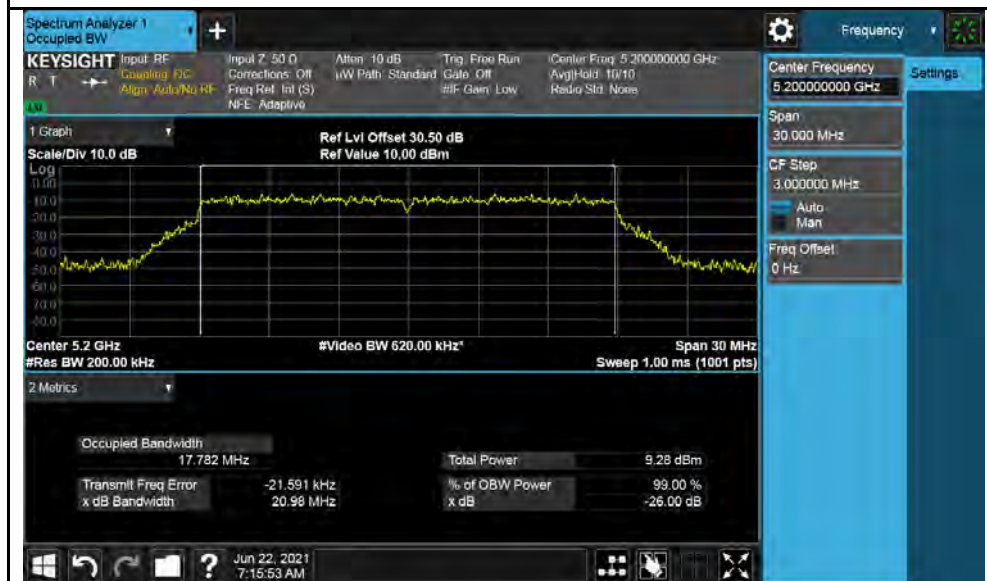
802.11a-5200MHz
