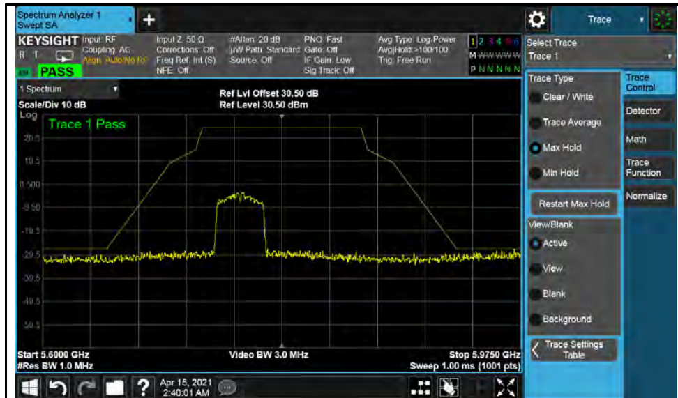
802.11n(HT40)-5755MHz
