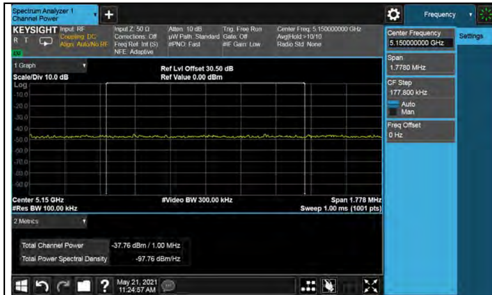
802.11ac(VHT20)-5180MHz
