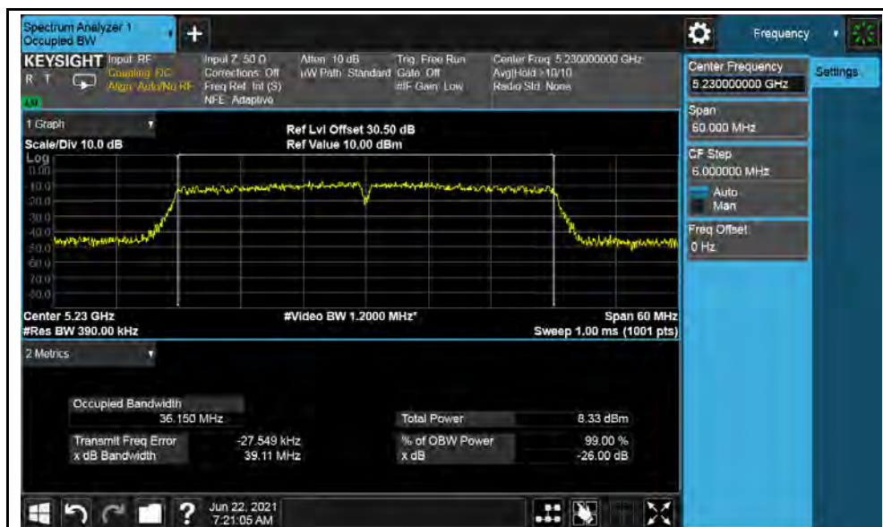
802.11ac-VHT40-5230MHz
