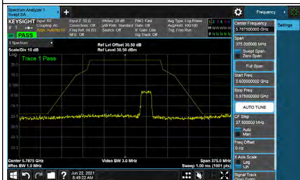
802.11ac (VHT20) – 5825MHz
