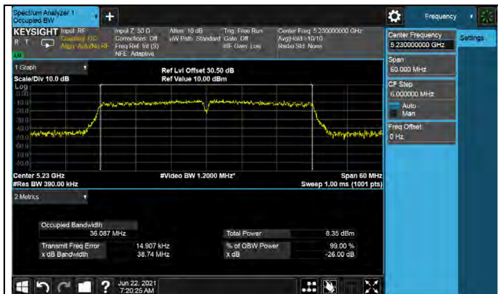
802.11n-HT40-5230MHz
