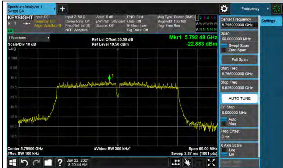
802.11ac-VHT40-5795MHz
