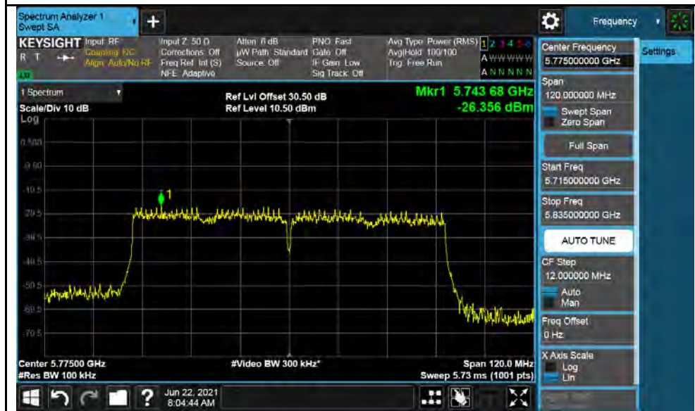
802.11ac-HT80-5775MHz
