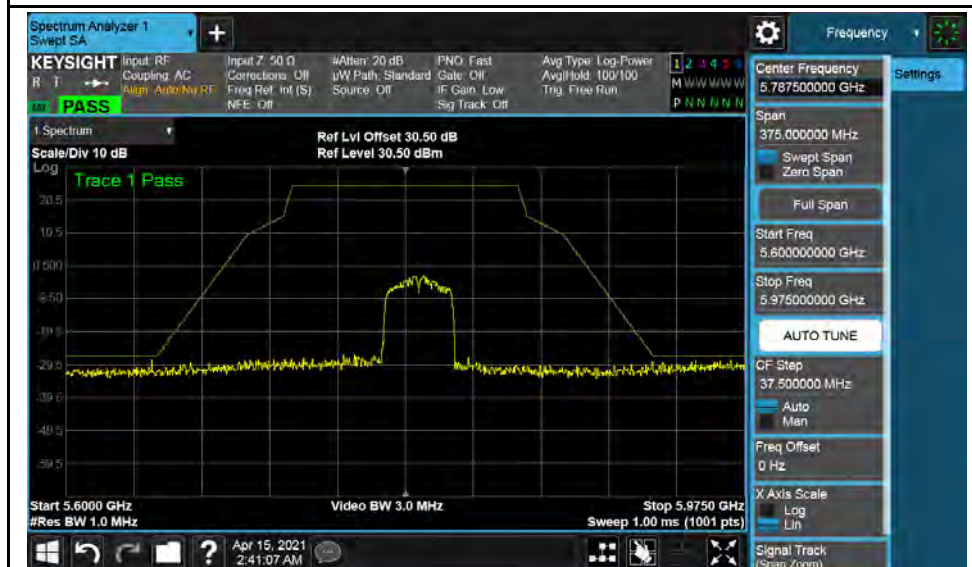
802.11n(HT40)-5795MHz
