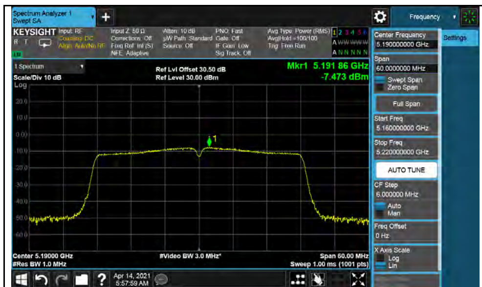
802.11n-HT40-5190MHz
