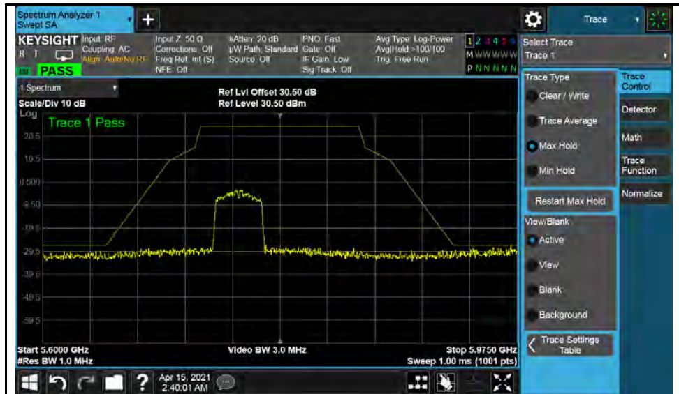
802.11n(HT40)-5755MHz
