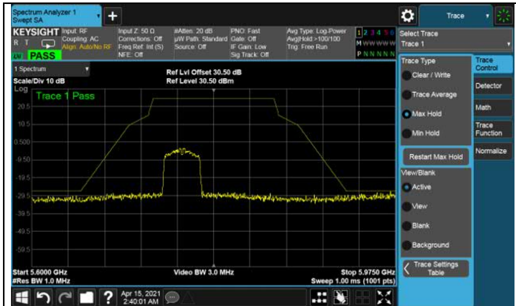
802.11n(HT40)-5755MHz
