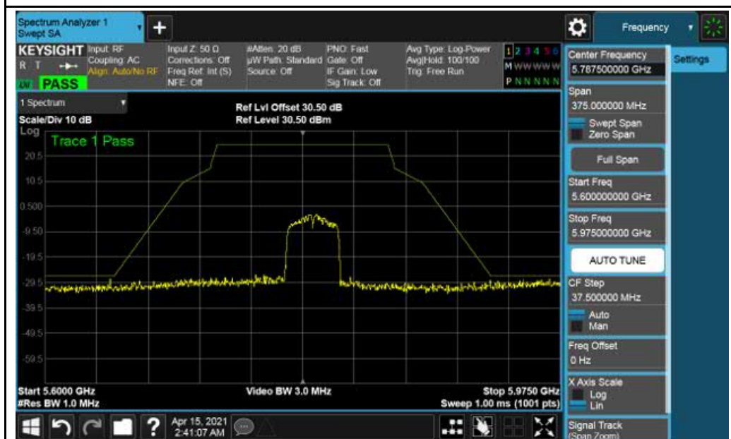
802.11n(HT40)-5795MHz
