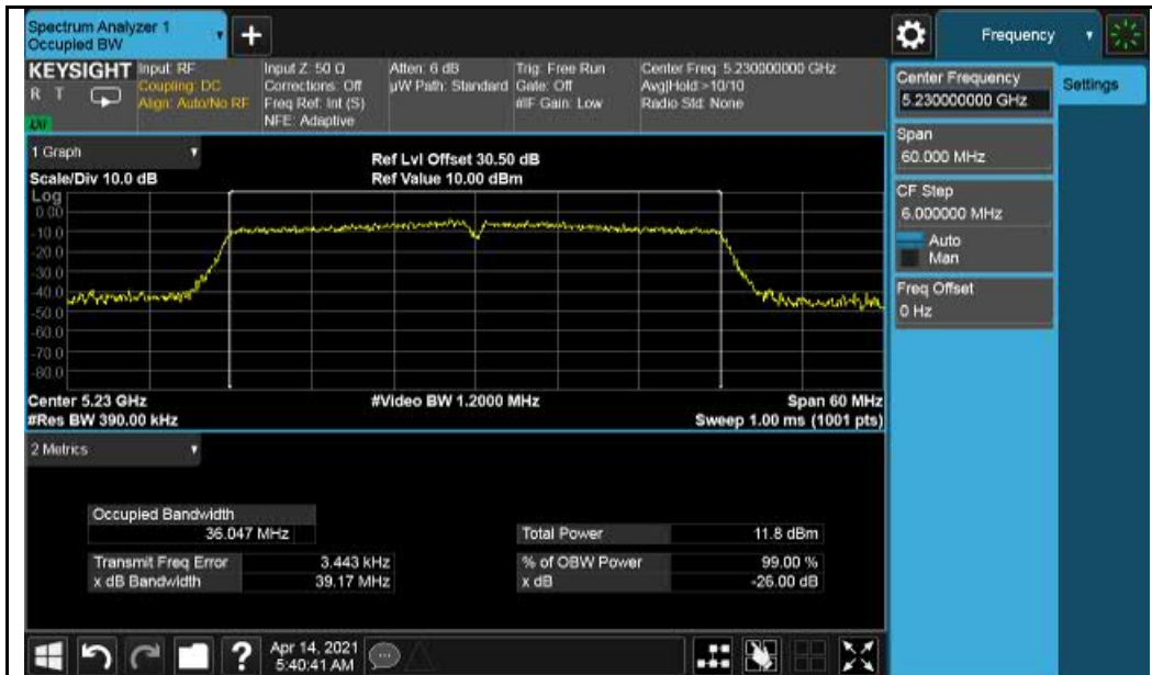
802.11n-HT40-5230MHz
