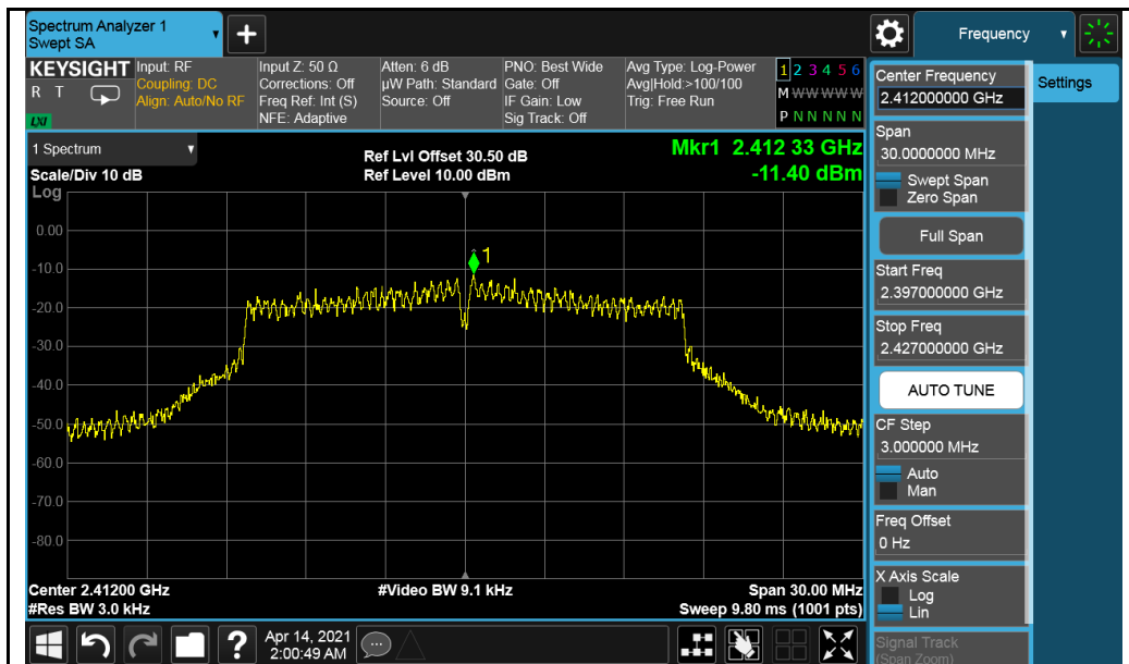
2412MHz
