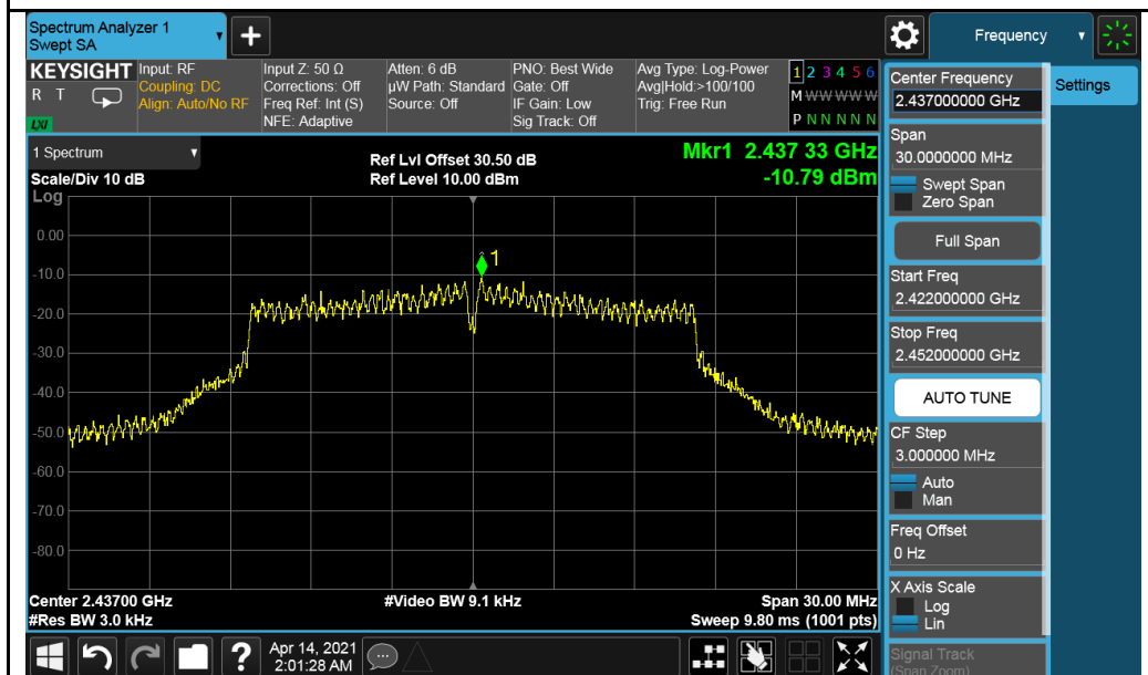
2437MHz
