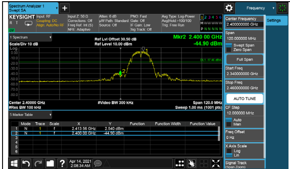
802.11b-2412MHz
