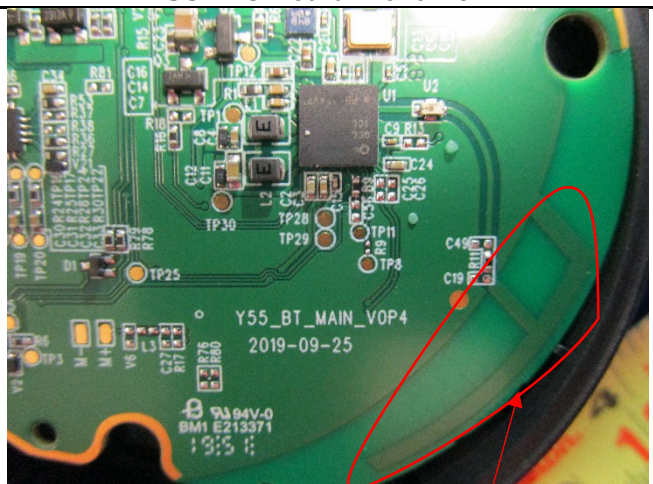
Antenna
