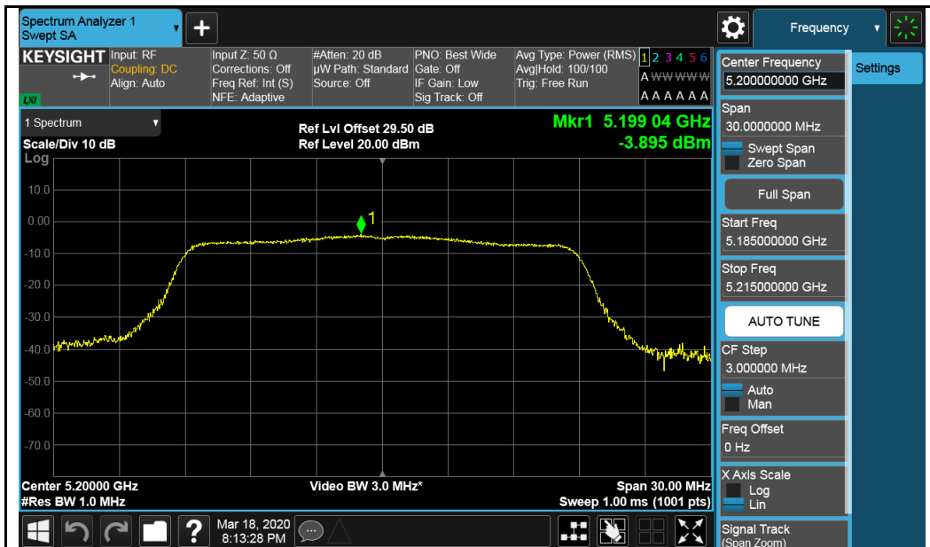
802.11n-HT20-5200MHz
