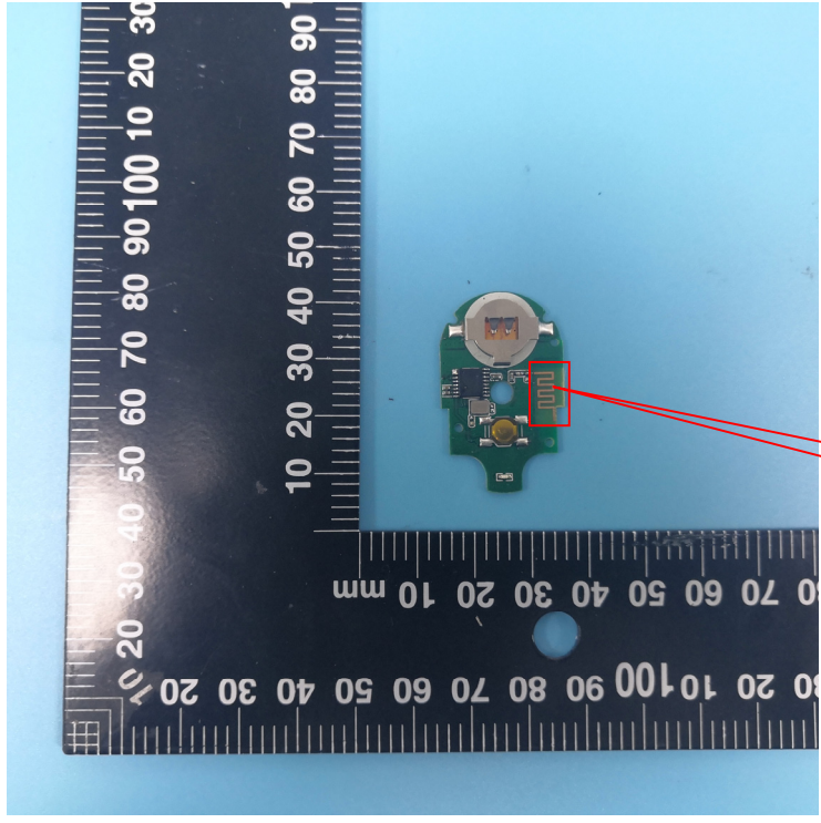
BLE Antenna
