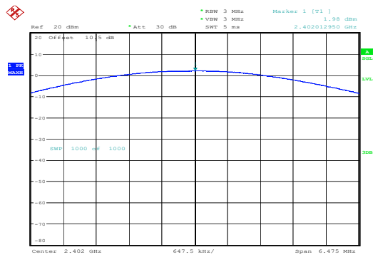
\pi/4 -DQPSK_Low 1.98dBm
