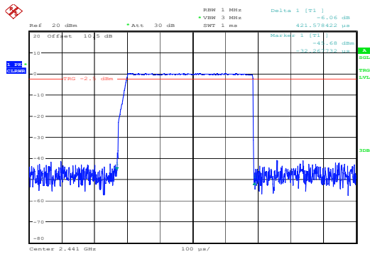
GFSK_Hopping_DH1 0.422ms
