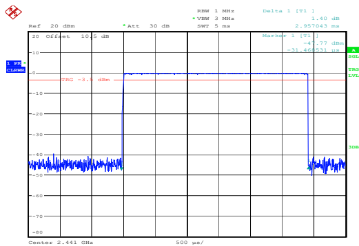
GFSK_Hopping_DH5 2.957ms
