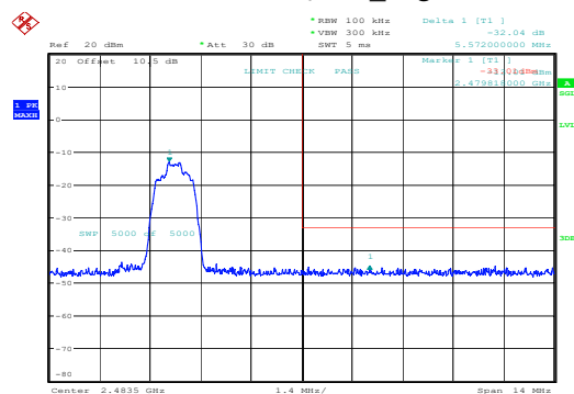
\pi/4 -DQPSK_High
