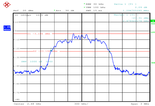
\pi/4 -DQPSK_High 1.295MHz
