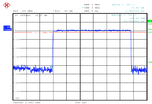
\pi/4 -DQPSK_Hopping_2DH5 2.962ms
