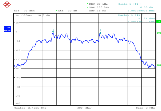
\pi/4 -DQPSK_Low 1.001MHz
