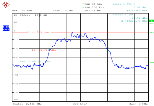
\pi/4 -DQPSK_Middle 1.289MHz
