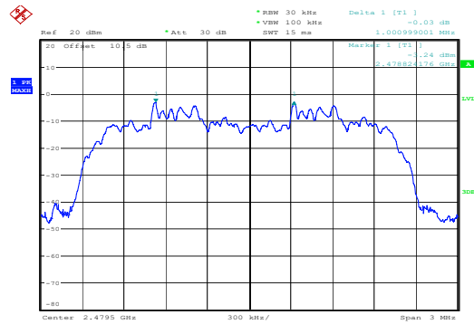
\pi/4 -DQPSK_High 1.001MHz
