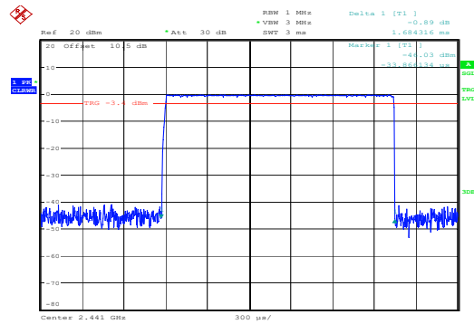
GFSK_Hopping_DH3 1.684ms
