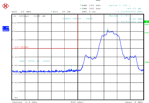
\pi/4 -DQPSK_Low
