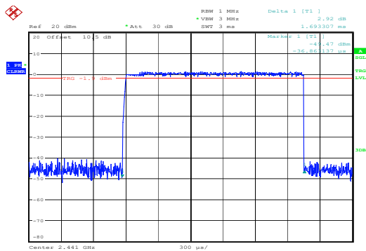
\pi/4 -DQPSK_Hopping_2DH3 1.693ms
