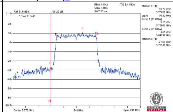
802.11ac(VHT80)_Chain3 / CH155
