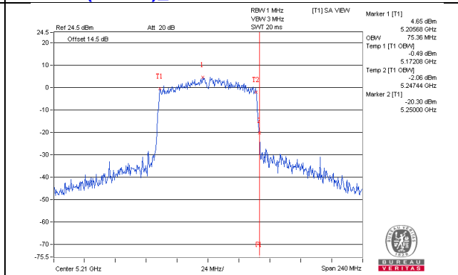
802.11ac(VHT80)_Chain3 / CH42
