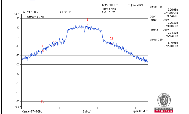
802.11a_Chain2 / CH149
