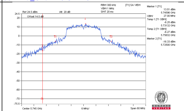
802.11a_Chain3 / CH149
