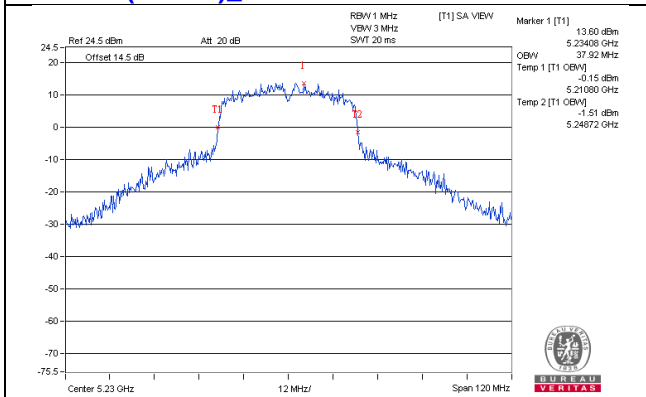
802.11ac (VHT40)_Chain3 / CH46
