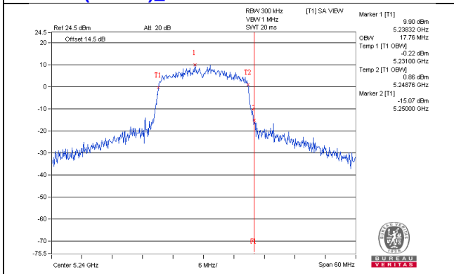
802.11ac(VHT20)_Chain2 / CH48
