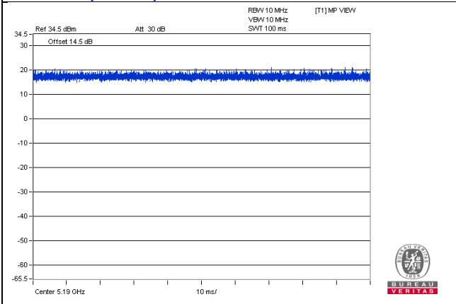
802.11ac (VHT40)
