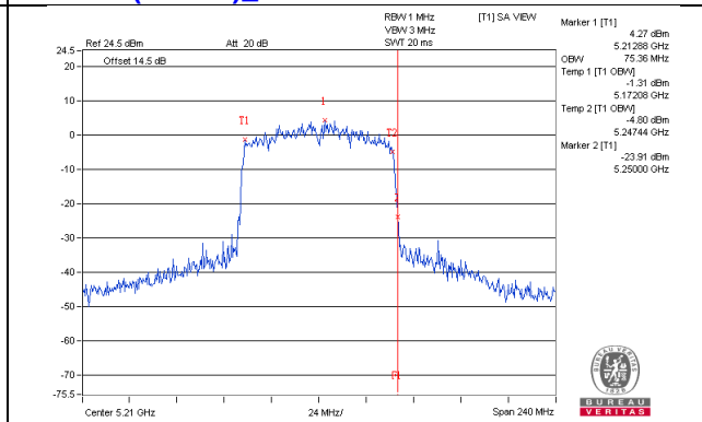
802.11ac(VHT80)_Chain3 / CH42
