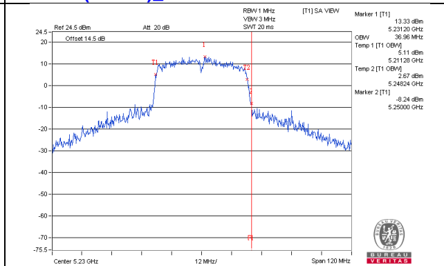
802.11ac(VHT40)_Chain3 / CH46
