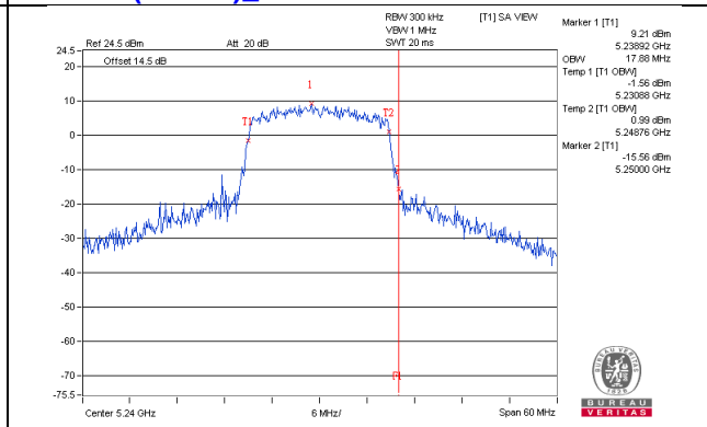
802.11ac(VHT20)_Chain3 / CH48
