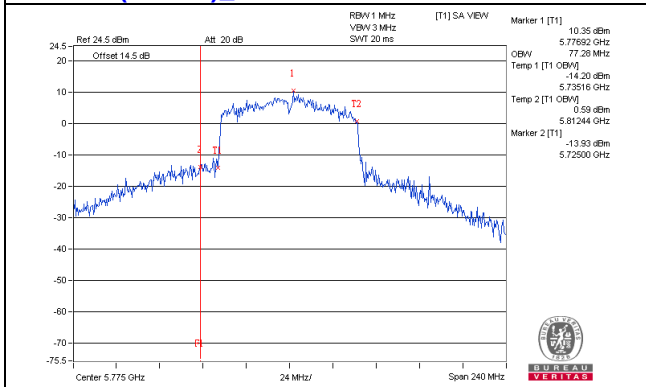
802.11ac(VHT80)_Chain2 / CH155
