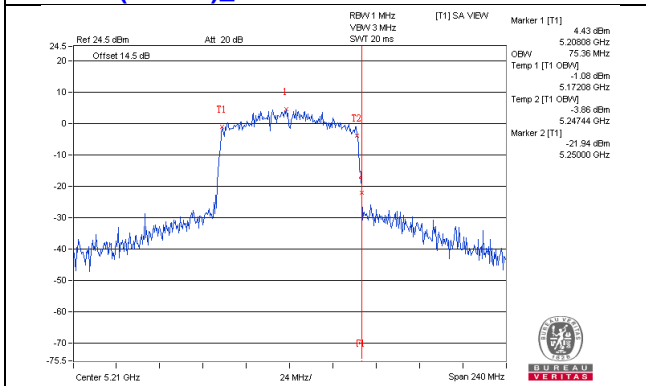
802.11ac(VHT80)_Chain2 / CH42
