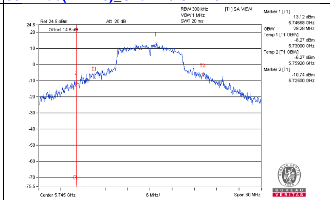
802.11ac(VHT20)_Chain3 / CH149
