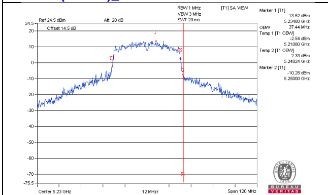
802.11ac(VHT40)_Chain2 / CH46
