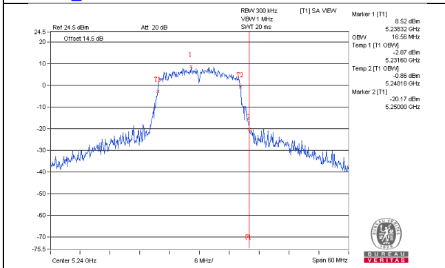
802.11a_Chain2 / CH48
