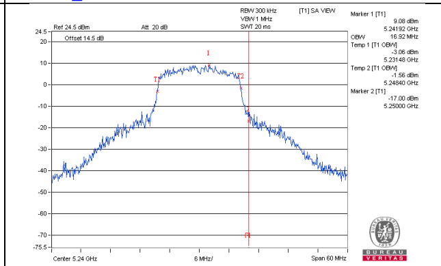
802.11a_Chain3 / CH48
