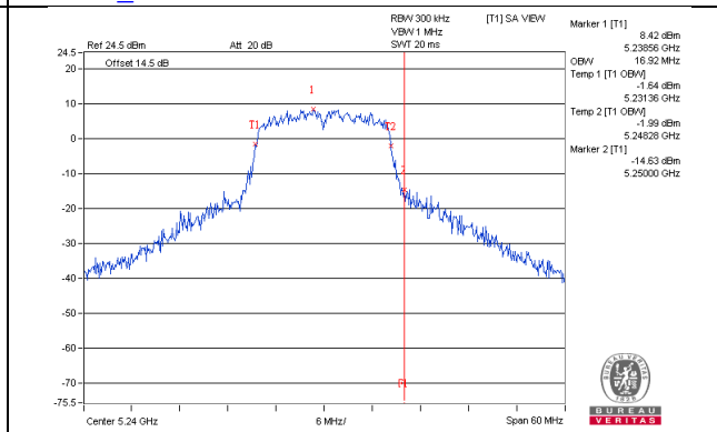
802.11ac(VHT20)_Chain1 / CH48
