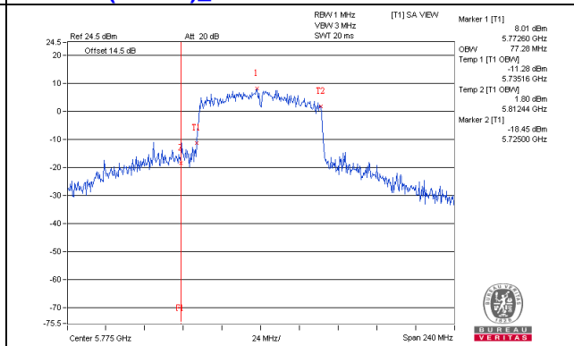
802.11ac(VHT80)_Chain3 / CH155
