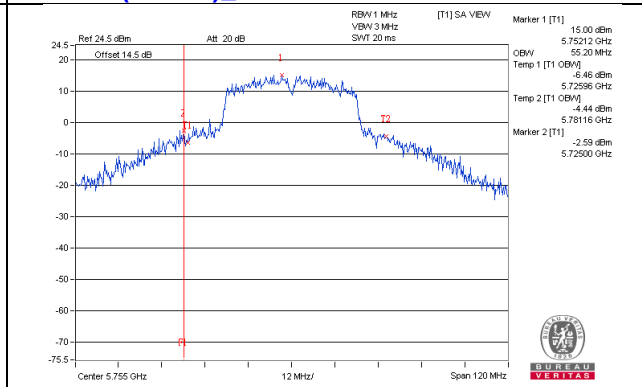
802.11ac(VHT40)_Chain3 / CH151
