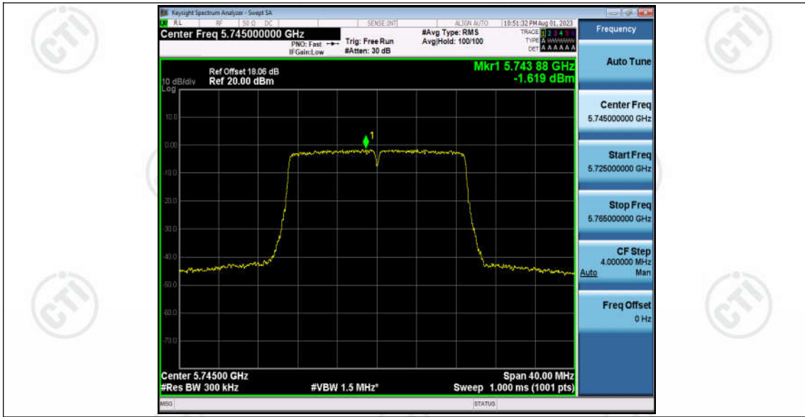
11N20MIMO_Ant2_5745
