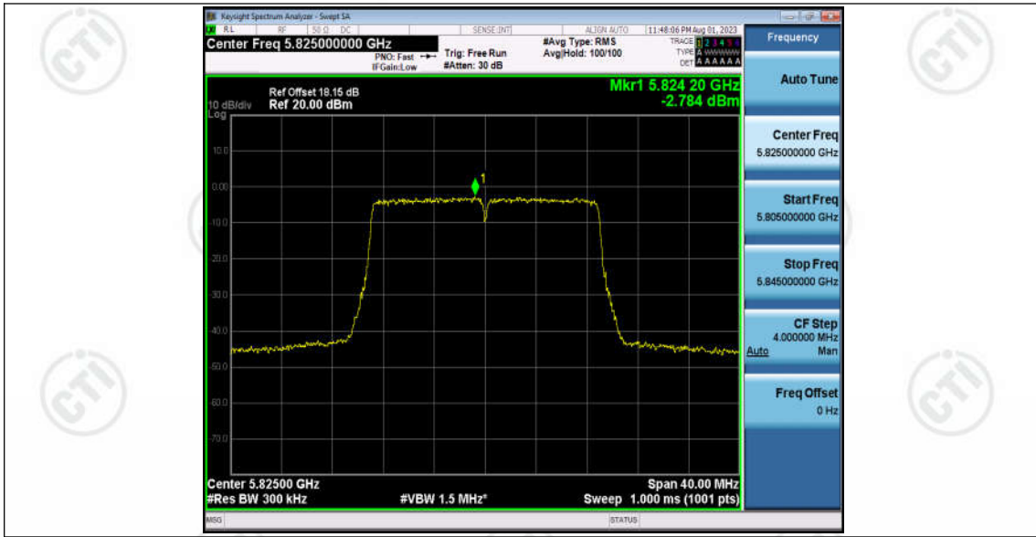
11AC20MIMO_Ant2_5825
