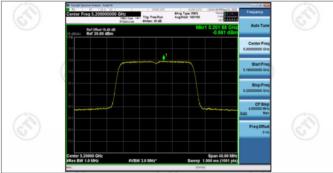
11N20MIMO_Ant2_5200
