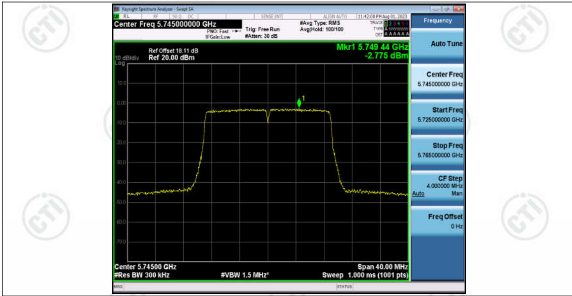
11AC20MIMO_Ant2_5745
