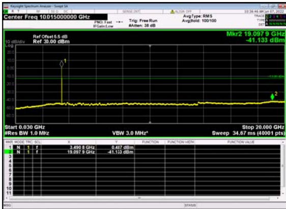
n77(20M)_DFT-s-OFDM_QPSK_ Edge_1RB_Left_633334_CH
