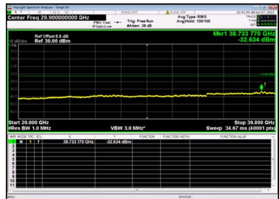
n77(20M)_DFT-s-OFDM_BPSK_ Edge_1RB_Left_636000_CH
