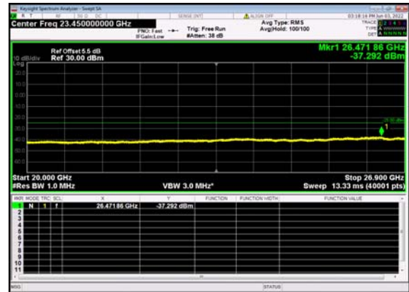
n41(90M)_DFT-s-OFDM_BPSK_ Edge_1RB_Left_Low_CH
