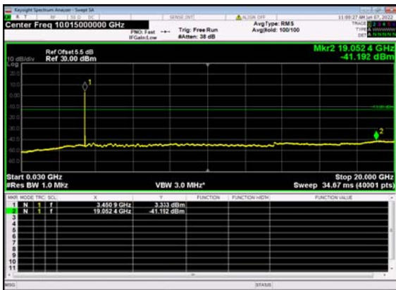
n77(30M)_DFT-s-OFDM_BPSK_ Edge_1RB_Left_631000_CH
