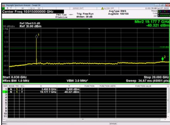
n77(30M)_DFT-s-OFDM_QPSK_ Edge_1RB_Left_631000_CH
