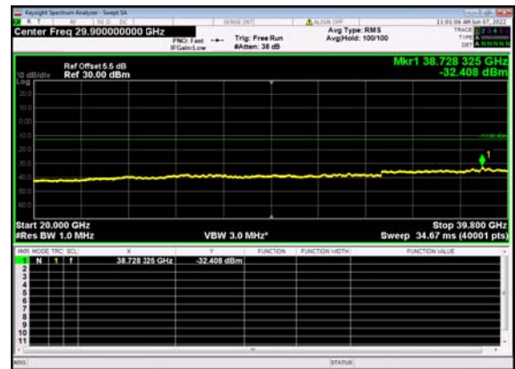
n77(30M)_DFT-s-OFDM_BPSK_ Edge_1RB_Left_631000_CH
