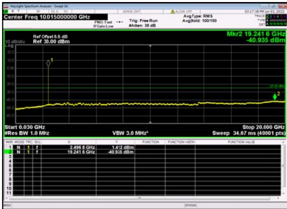
n41(90M)_DFT-s-OFDM_BPSK_ Edge_1RB_Left_Low_CH
