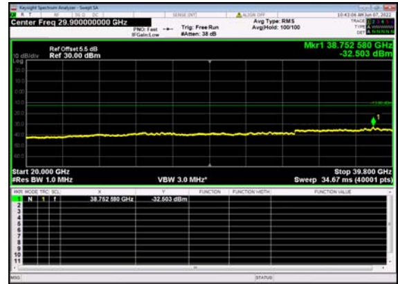
n77(20M)_DFT-s-OFDM_QPSK_ Edge_1RB_Left_636000_CH
