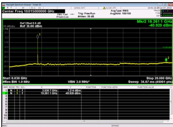
n77(20M)_DFT-s-OFDM_BPSK_ Edge_1RB_Left_636000_CH
