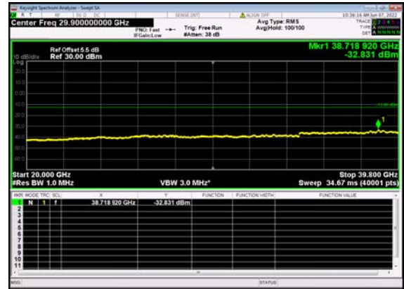
n77(20M)_DFT-s-OFDM_BPSK_ Edge_1RB_Left_633334_CH
