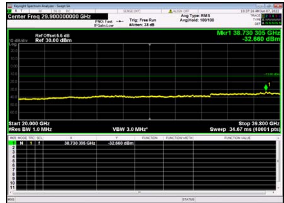
n77(20M)_DFT-s-OFDM_QPSK_ Edge_1RB_Left_633334_CH
