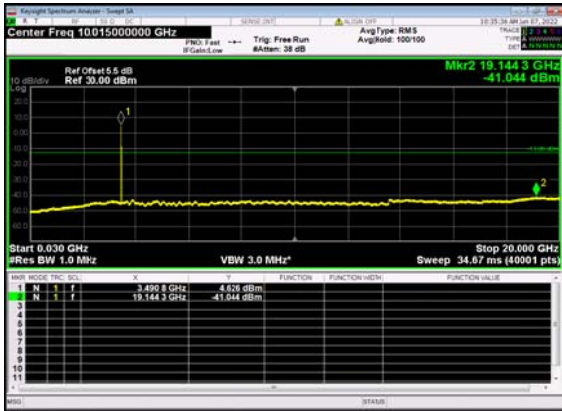
n77(20M)_DFT-s-OFDM_BPSK_ Edge_1RB_Left_633334_CH
