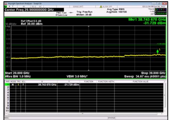
n77(60M)_DFT-s-OFDM_BPSK_ Edge_1RB_Left_Low_CH
