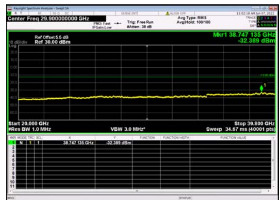
n77(30M)_DFT-s-OFDM_QPSK_ Edge_1RB_Left_631000_CH
