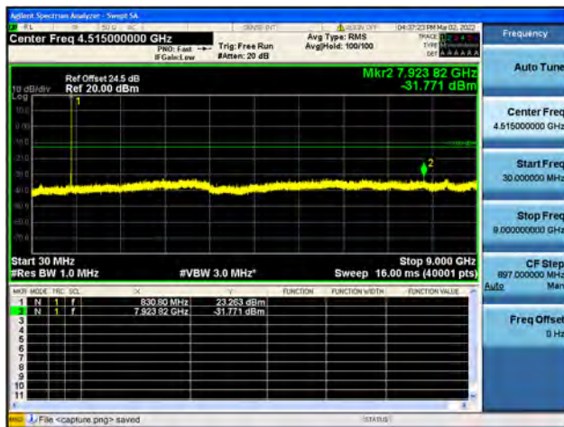
Band19 / 10MHz / Low CH / 64QAM
