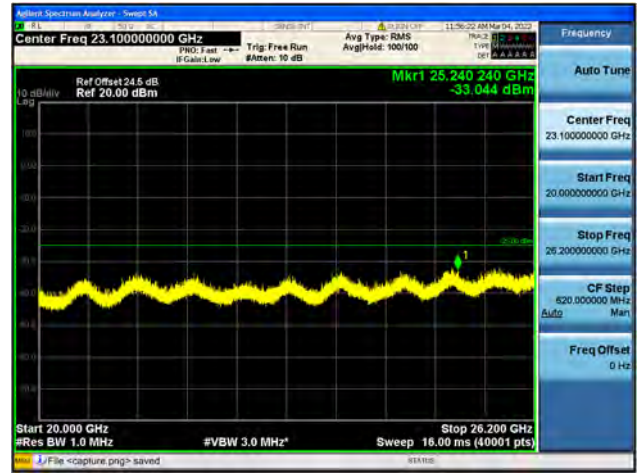
Band38 / 20MHz / Low CH / 16QAM
