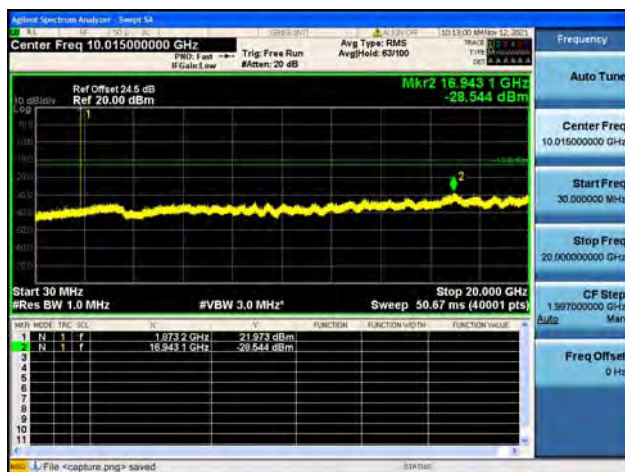
Band2 / 15MHz / Mid CH / 64QAM
