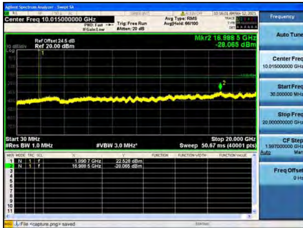
Band2 / 20MHz / High CH / 64QAM
