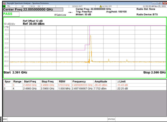
N41(50M)_DFT-s-OFDM_BPSK_Edge_1RB_Left_Low
