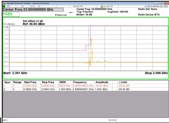
N41(20M)_DFT-s-OFDM_BPSK_Edge_1RB_Left_Low
