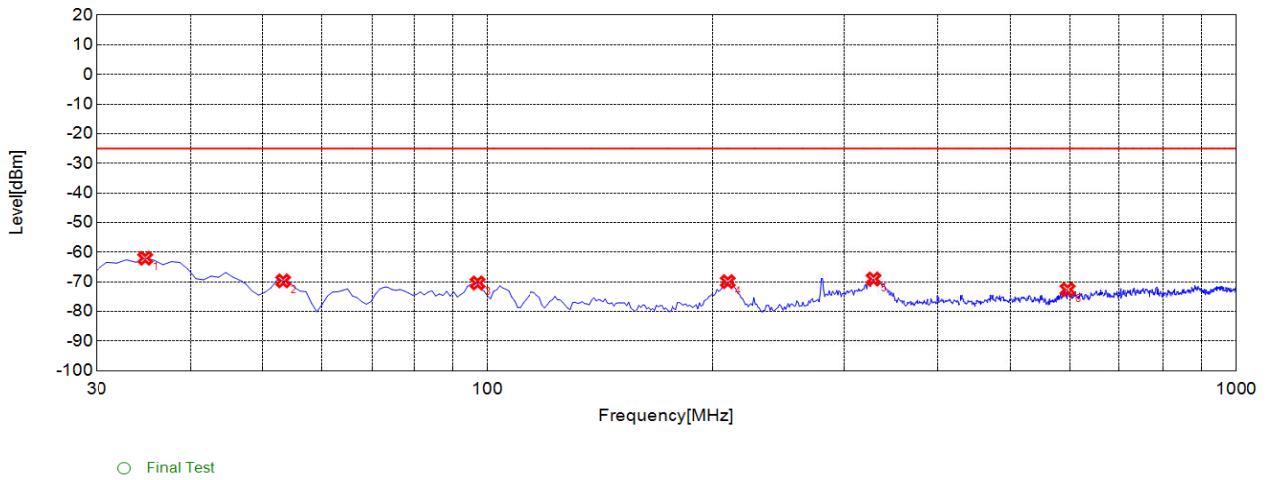
n41 503202 40Mhz CP-OFDM 16 QAM 1RB_Right 30M-1G V
