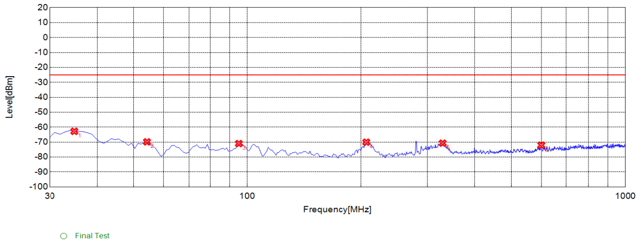
n41 518598 40Mhz CP-OFDM 16 QAM 1RB_Right 30M-1G V
