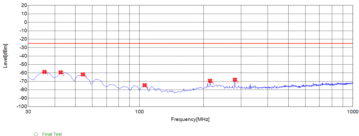
n41 503202 40Mhz CP-OFDM 16 QAM 1RB_Right 30M-1G H
