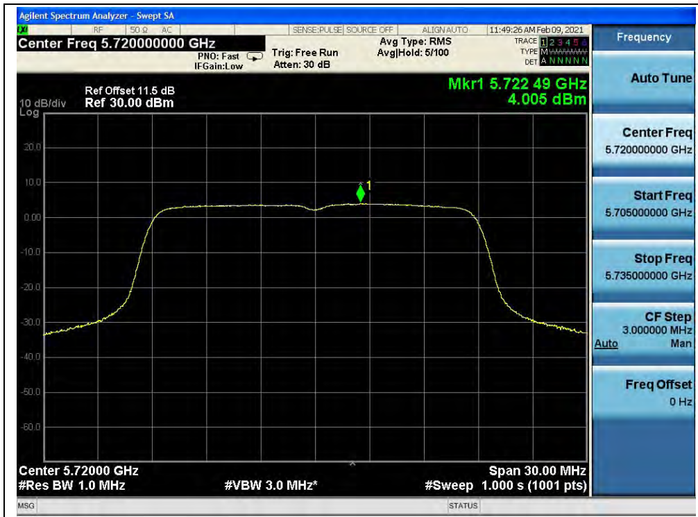
(Channel 144, 5720MHz, 802.11n (HT20), ANT0)
