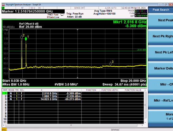
B2_N41(60M)_DFT-s-OFDM_QPSK_Edge_ 1RB_Left_Low_CH
