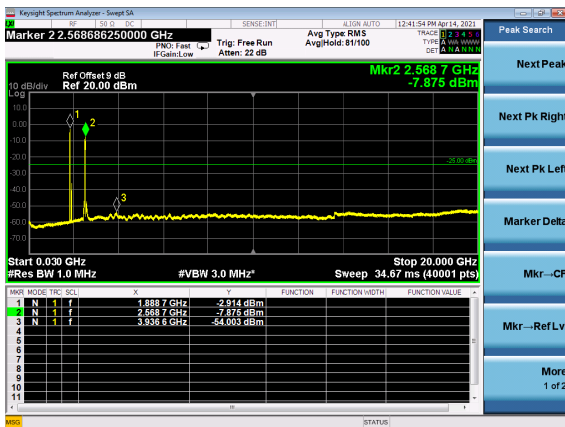
B2_N41(60M)_DFT-s-OFDM_BPSK_Edge_ 1RB_Left_Low_CH
