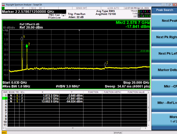
B2_N41(50M)_DFT-s-OFDM_BPSK_Edge_ 1RB_Left_Mid_CH
