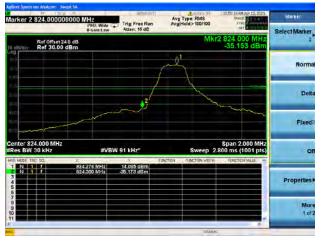
Band26 / 1.4MHz / High CH / QPSK / 1 RB
