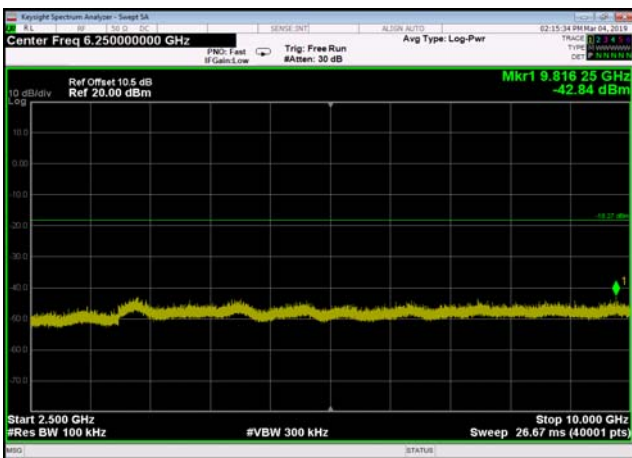
,Plot 4,2500MHz~10000MHz-802.11n(HT40),2452MHz,Ant0
