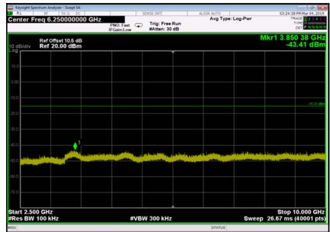
,Plot 4,2500MHz~10000MHz-802.11n(HT20),2437MHz,Ant1
