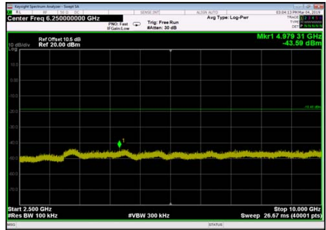
,Plot 4,2500MHz~10000MHz-802.11n(HT40),2437MHz,Ant1
