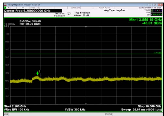
,Plot 4,2500MHz~10000MHz-802.11n(HT20),2462MHz,Ant1
