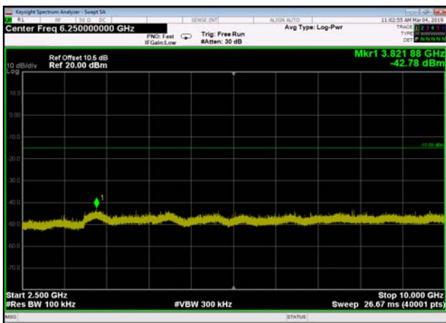
,Plot 4,2500MHz~10000MHz-802.11n(HT20),2462MHz,Ant0
