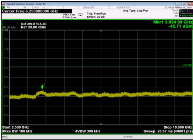
,Plot 4,2500MHz~10000MHz-802.11n(HT40),2437MHz,Ant0
