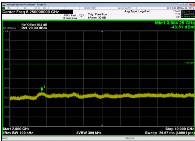
,Plot 4,2500MHz~10000MHz-802.11n(HT20),2437MHz,Ant0
