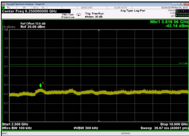
,Plot 4,2500MHz~10000MHz-802.11n(HT40),2452MHz,Ant0
