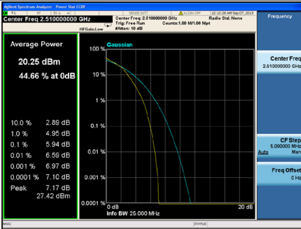
20MHz/16QAM / MCH
