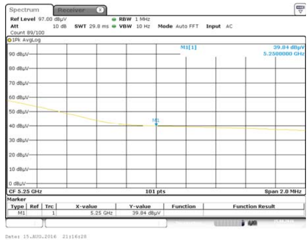
Band I 11a(HT20) CH44, AV
