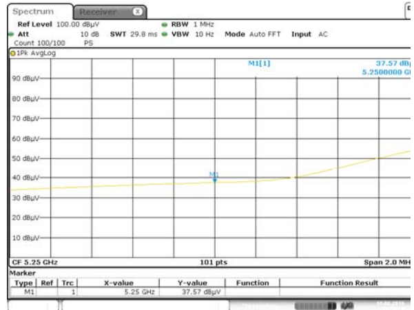
Band II 11a(HT20) CH52, AV
